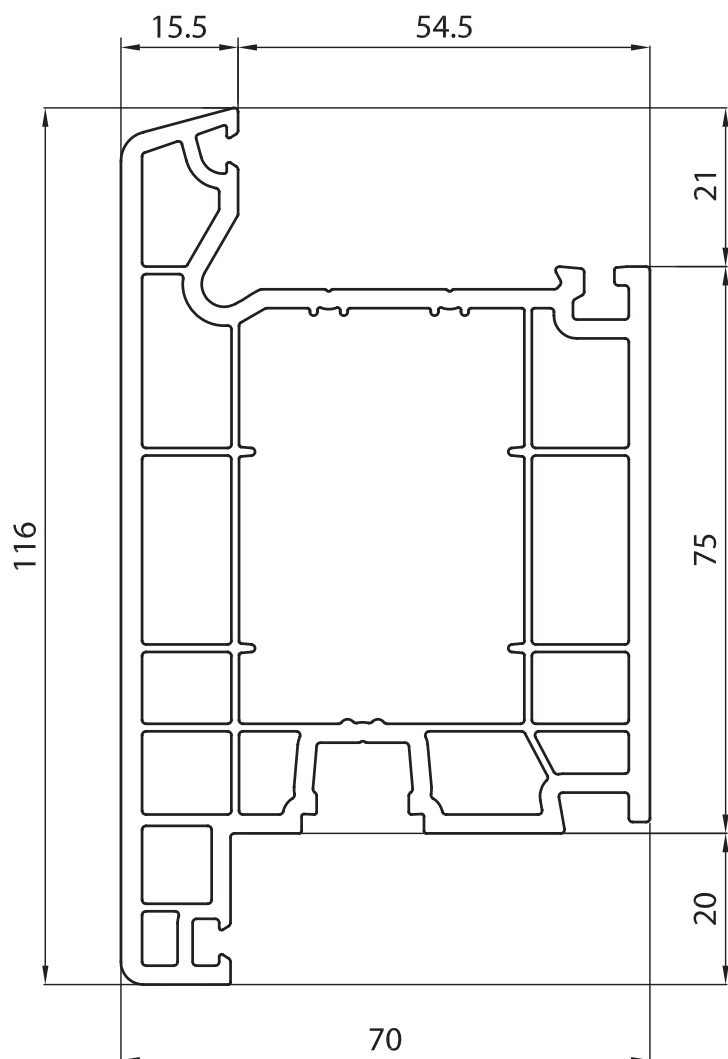
Дверная створка (наружного открывания) Арт. TD 70/116
