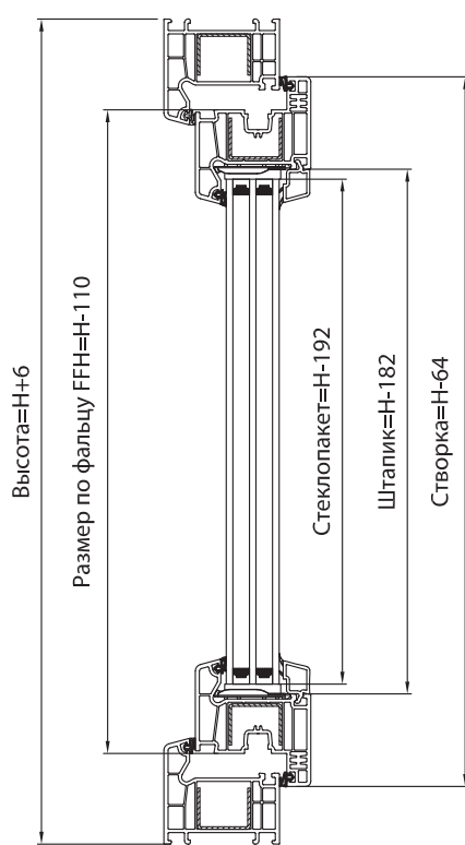
Сечение Н-Н
