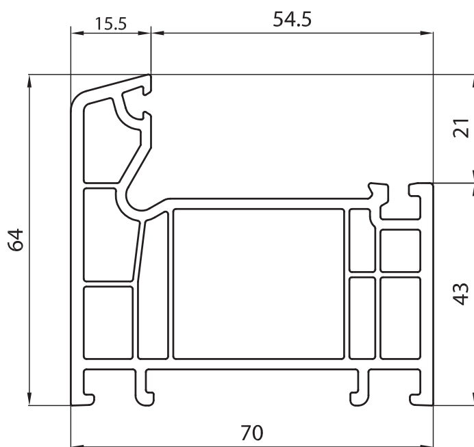
Рама Арт. TL 70/64
