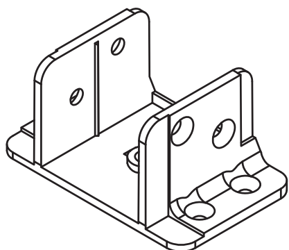
Мех. соединитель металлический Арт. TT 82 M
