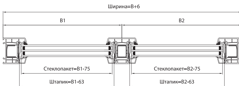
Сечение В-В
