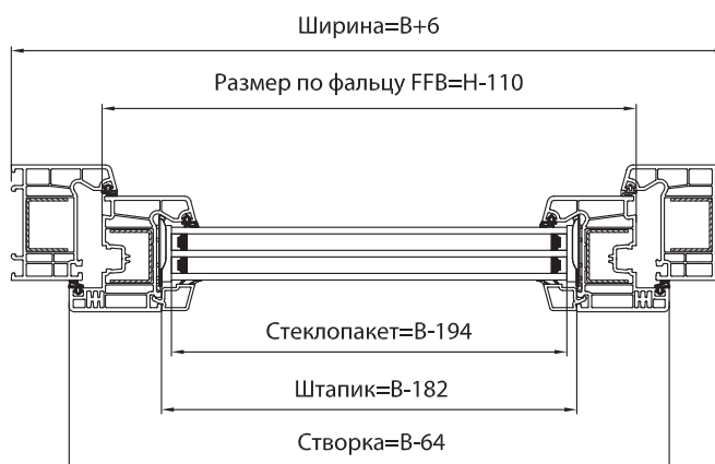
Сечение В-В
