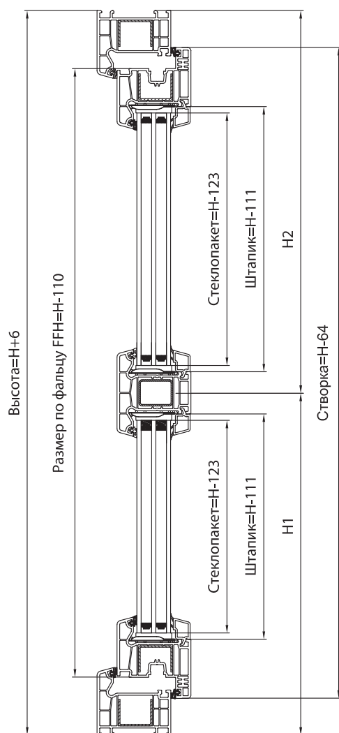
Сечение Н-Н
