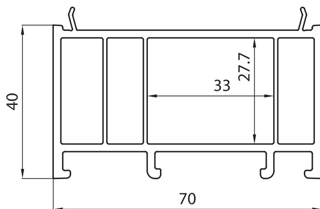
Расширитель 40 мм Арт. PE 608/70
