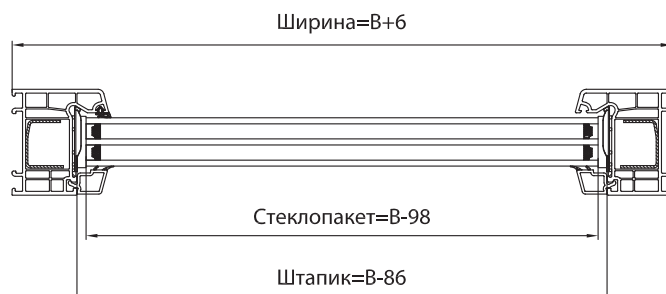
Сечение В-В
