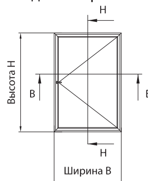
Одностворчатое окно
