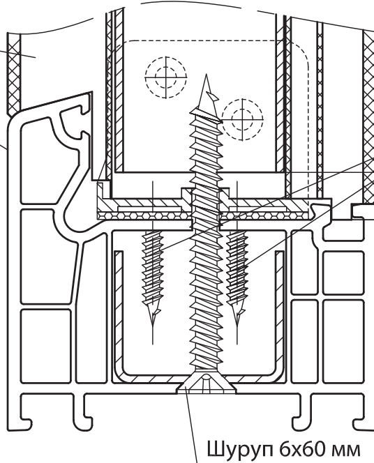
Шуруп 3.9x25 потайн. гол. 4 шт.
