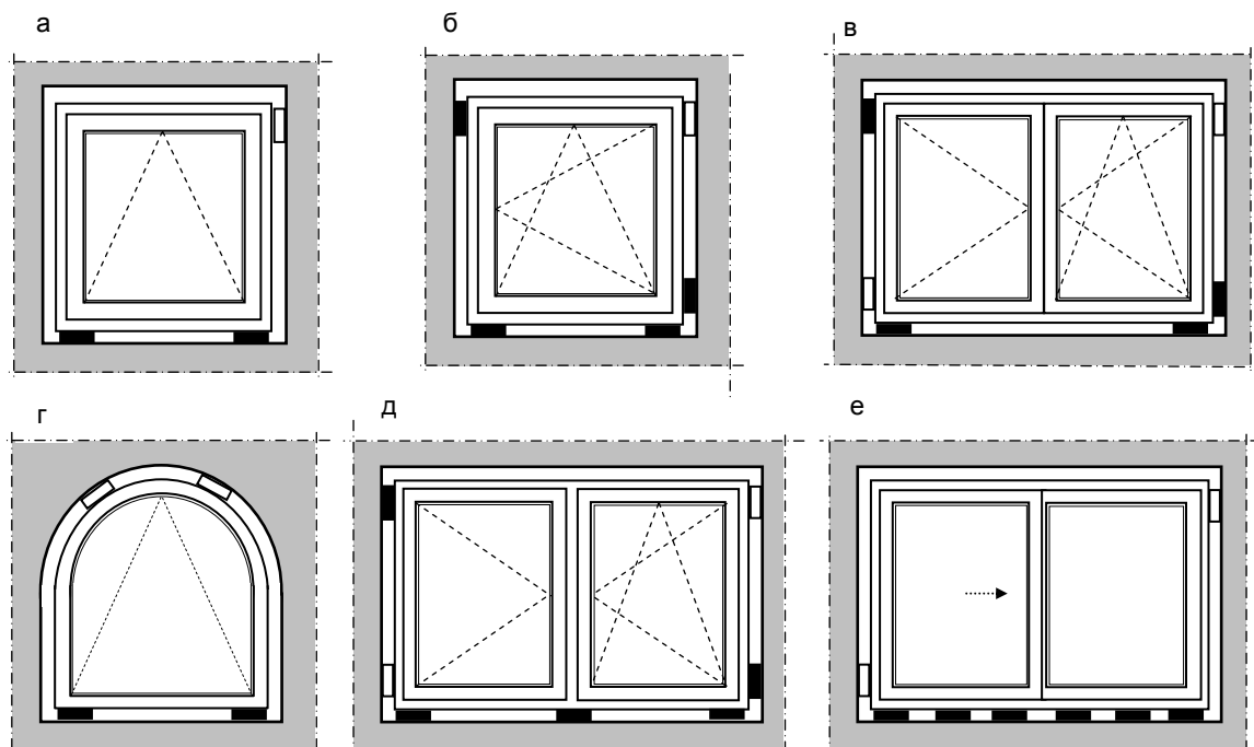
Рис.7.2. Схемы размещения несущих и дистанционных колодок оконных блоков различной конфигурации при различных способах открывания створок: а, д – откидным; б, в, г – поворотно-откидным; е – раздвижным ( ■ - несущие колодки, □ - дистанционные колодки )
