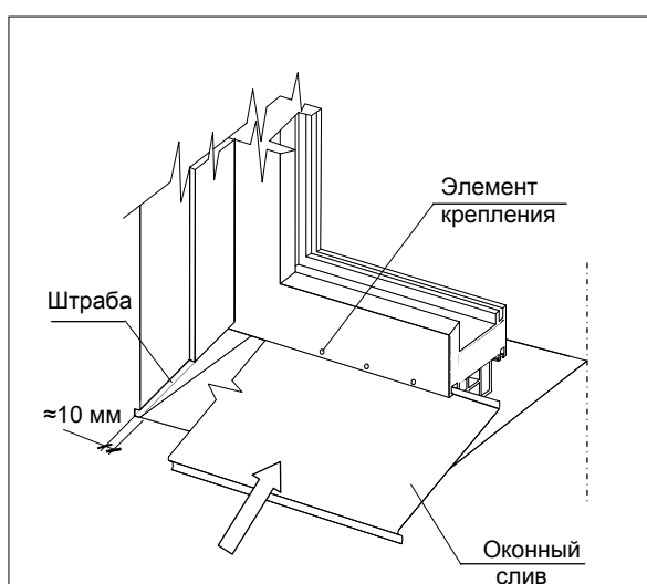
Схема установки оконного слива
