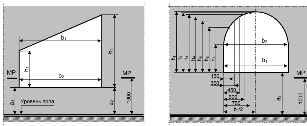
Рис.5.4. Схемы замеров оконных проемов непрямоугольной конфигурации
