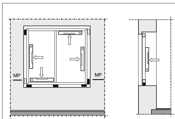
Схема проверки вертикальности установки оконного блока)
