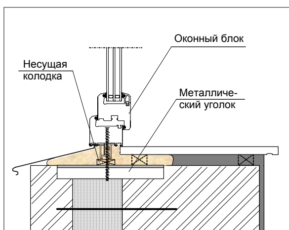
Схема передачи нагрузки от оконного блока на наружную стену
