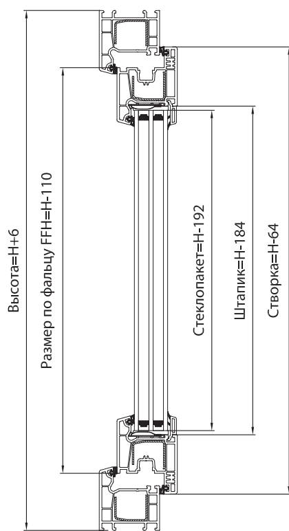
Сечение Н-Н
