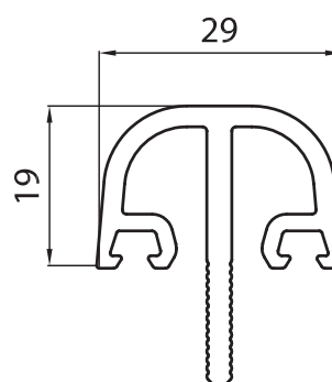
Крышка статического соединителя Арт. PS 609
