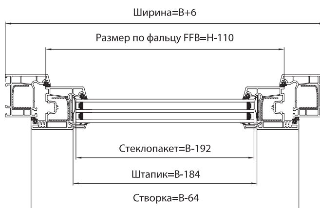
Сечение В-В
