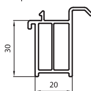
Подставочный профиль Арт. PW 58
