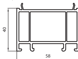
Расширитель 40 мм Арт. PE 607/58
