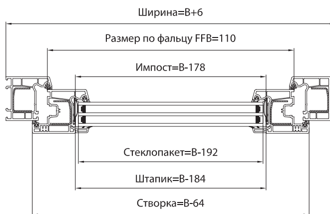
Сечение В-В
