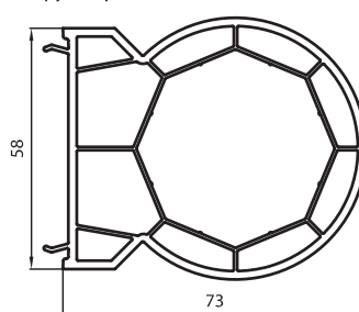
Труба Арт. PP 614/58
