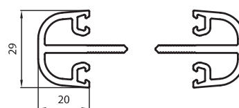
Крышка статического соединителя Арт. PS 609
