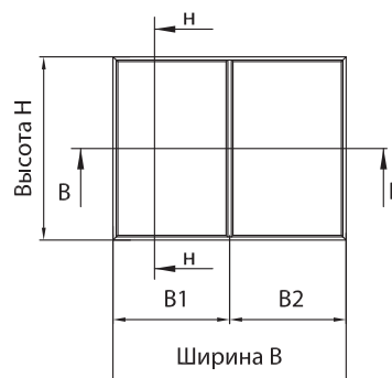
Глухое окно с импостом
