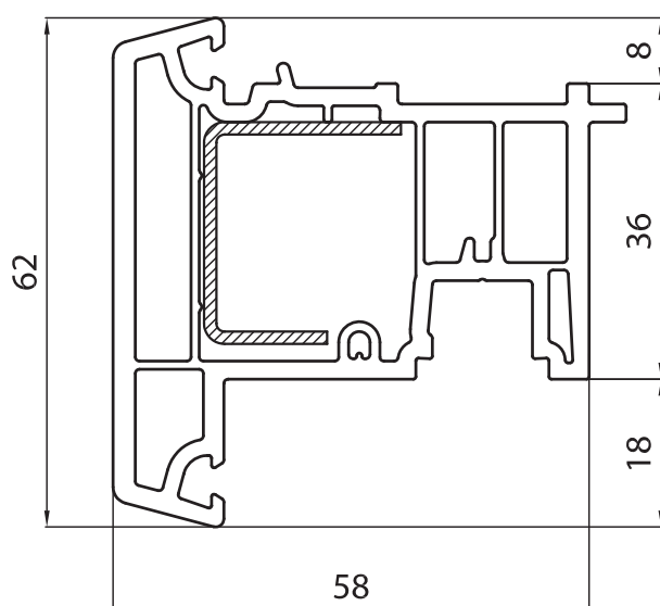
Штульп Арт. CS 58/62
