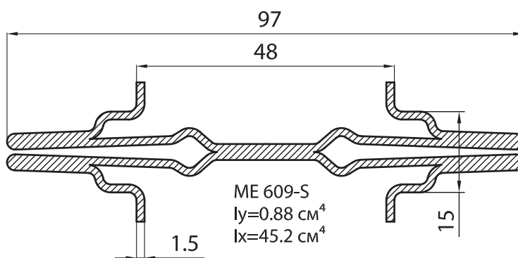
Металлопрофиль статический MP 609-S
