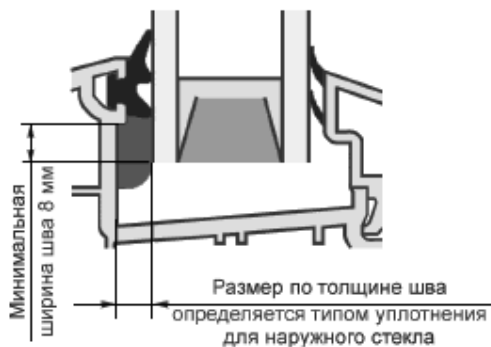
Рисунок 2 - Пример конструкции узла вклейки стеклопакета
