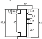
Профиль стыковочный Арт. С640/30X
