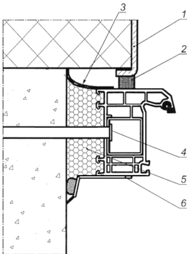
Рисунок А.6 - Узел бокового примыкания оконного блока к проему с четвертью в стене из ячеистобетонных блоков (плотностью 400-450 \text{ кг/м}^3 ) с облицовкой кирпичом и отделкой внутреннего откоса панелью
