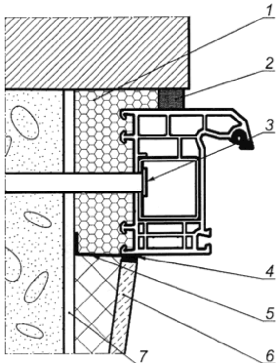
1- пенный утеплитель; 2- изоляционная саморасширяющаяся паропроницаемая лента (ПСУЛ); 3- рамный дюбель; 4- герметик; 5- пароизоляционная лента; 6- панель отделки внутреннего откоса; 7- штукатурный выравнивающий слой внутреннего откоса
