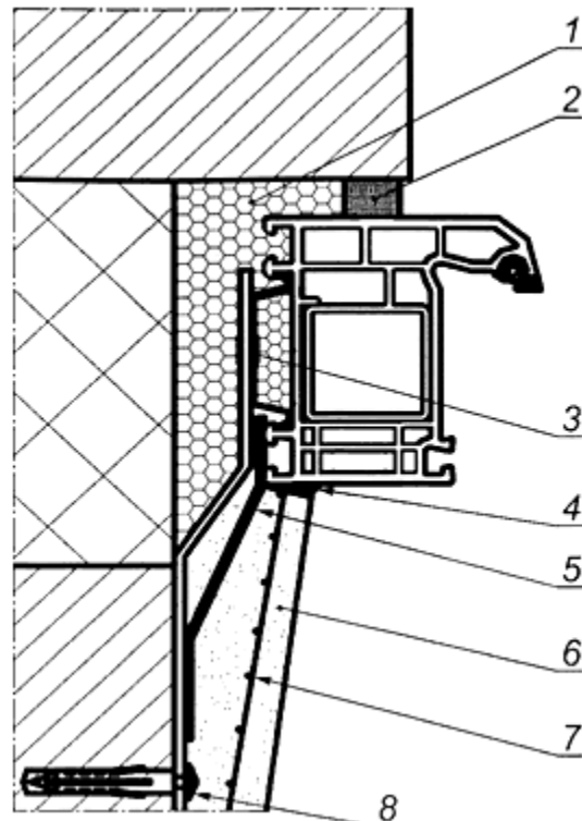
Рисунок А.2 - Узел бокового примыкания оконного блока к проему без четверти в стене из кирпича и с отделкой внутреннего откоса облицовочной панелью
