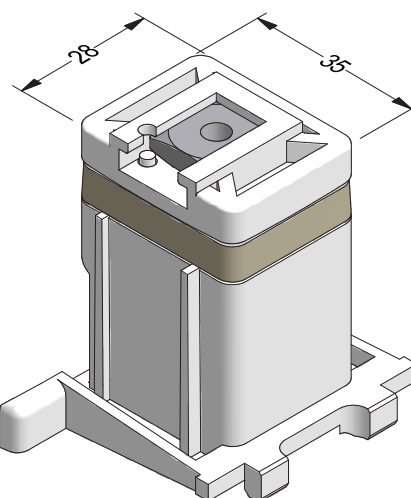
Механический соединитель импоста 86 с уплотняющей подушкой
