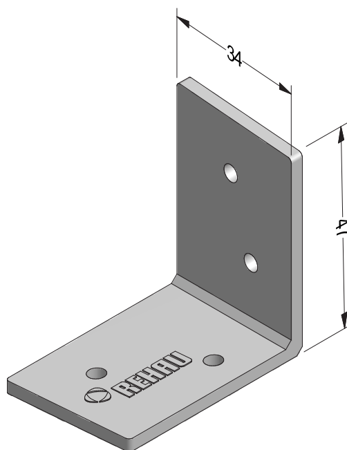
Литой ремонтный уголок универсальный
