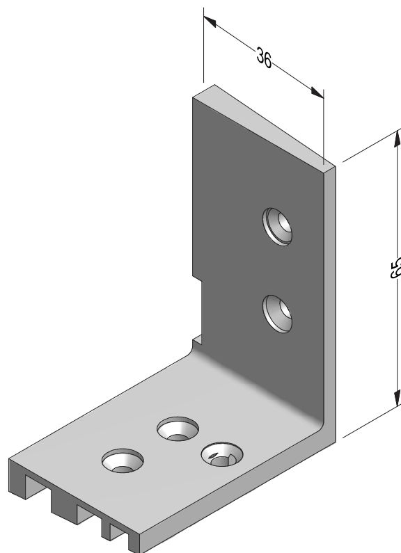
Литой уголок для установки стеклоделаящих горбыльков в створку
