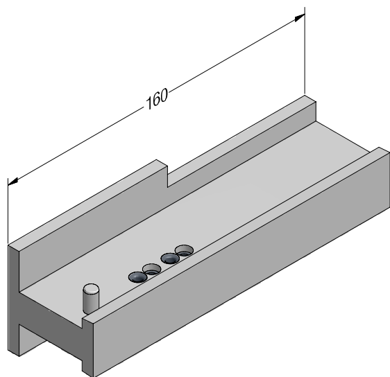
Шаблон импоста
