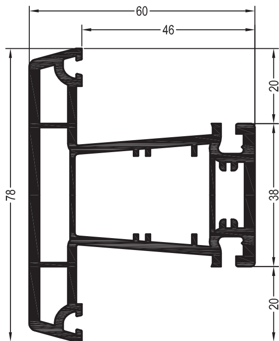
Профили импостов / поперечин
