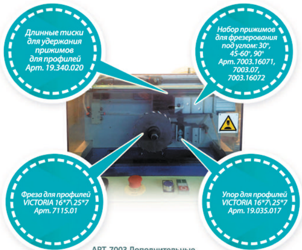
Арт. 7003 Дополнительные функциональные элементы к станку
