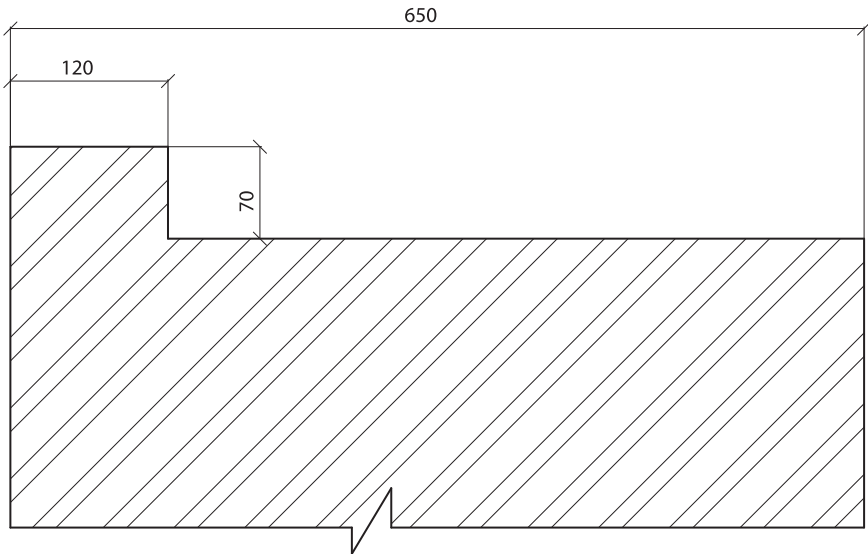
Рисунок К.3 – Эскиз участка ограждающей конструкции входящий в узел примыкания.
