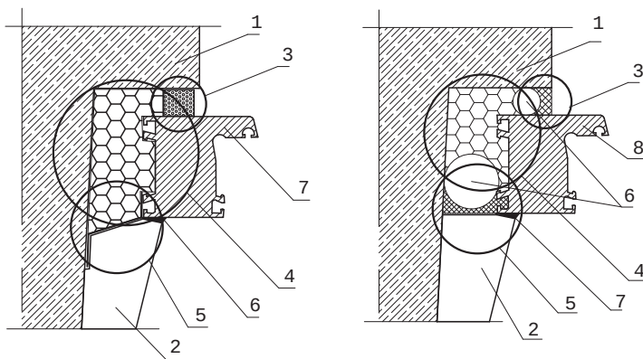
Рисунок 1 – Принципиальная схема узла примыкания к проемам с четвертью
