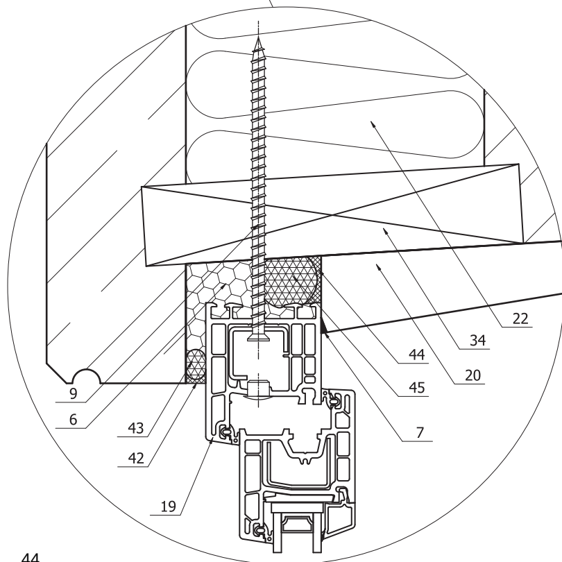
Рисунок А17 – Узел примыкания СПК к проему трехслойной железобетонной панели с эффективным утеплителем в качестве среднего слоя. Проем с четвертью. Внутренние откосы оштукатуриваются. Для герметизации монтажного шва применены мастичные герметики.
