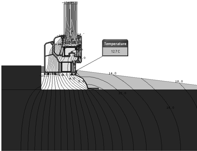
Рисунок К.7 – Температурное поле узла примыкания светопрозрачной конструкции из ПВХ профиля XXXXXXXXXXXXXXXXXX . Сечение узла примыкания вертикального бруска оконной коробки к ограждающей конструкции с четвертью. Откос выполнен цементно-песчаным раствором с последующей окраской. Температура на участке примыкания подоконника к коробке рамы 12,7 °С.
