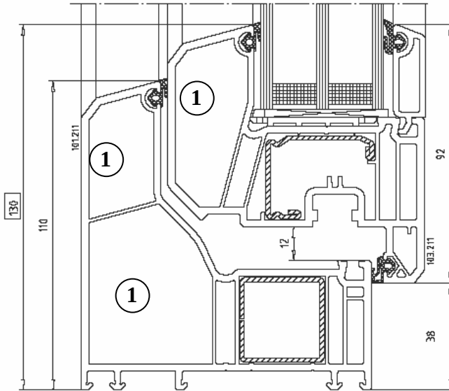
Рисунок К.1 – Конструкция коробка + створка светопрозрачной ограждающей конструкции XXXXXXXXXXXXXXXXXX (боковые и верхнее примыкания). Полости 1 заполнены экструдированным полистиролом.
