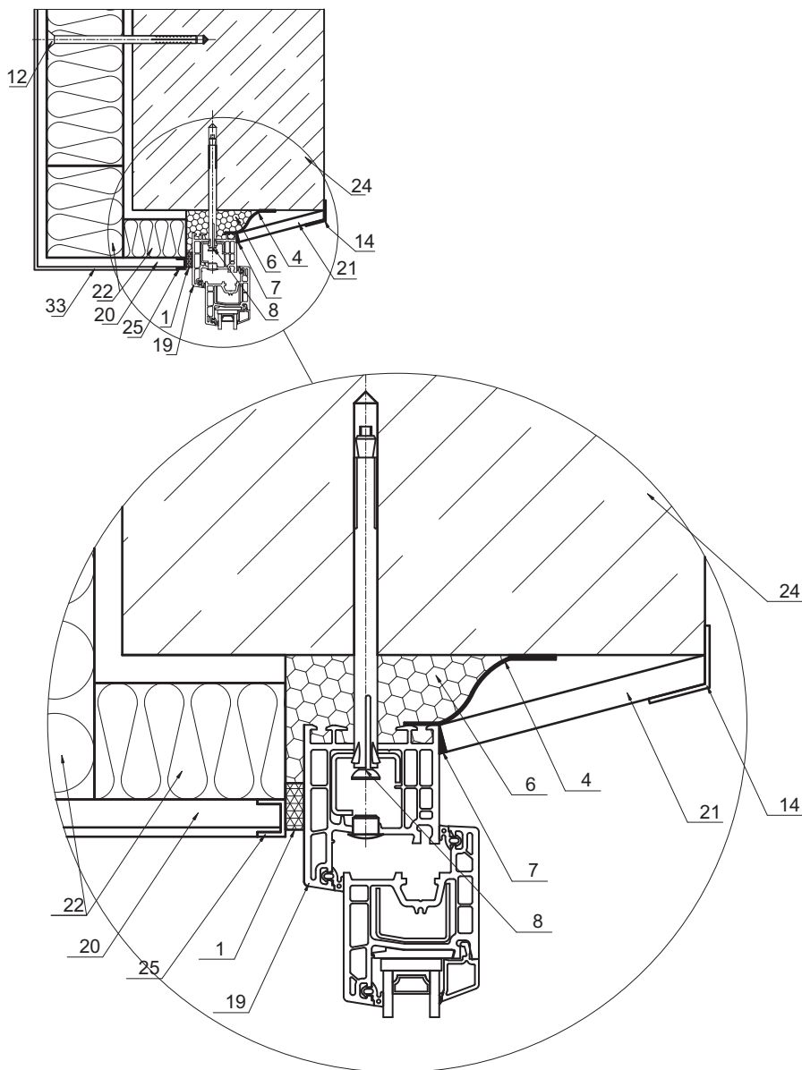
Рисунок А5 – Узел примыкания СПК к стене из железобетона и эффективного утеплителя со стороны улицы. Утеплитель в проеме образует четверть. СПК смещается на середину толщины несущей части стены. Внутренние откосы отделываются плитными материалами. Необходим теплотехнический расчет данного узла.
