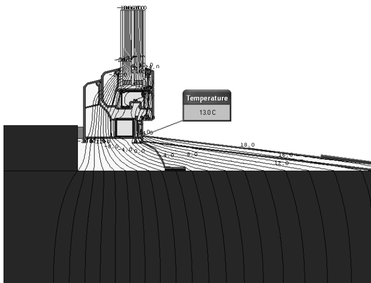
Рисунок К.10 – Температурное поле узла примыкания светопрозрачной конструкции из ПВХ профиля XXXXXXXXXXXXXXXXXX . Сечение узла примыкания вертикального бруска оконной коробки к ограждающей конструкции с четвертью. Откос выполнен ПВХ панелью толщиной 10 мм. С утеплением внутреннего откоса. Температура на участке примыкания подоконника к коробке рамы 13,0 °С.
