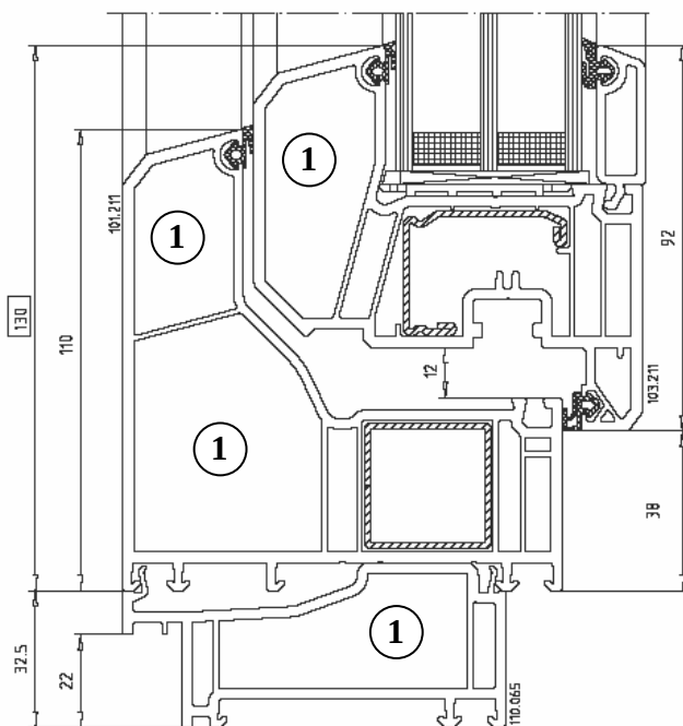
Рисунок К.2 – Конструкция коробка + створка + подставочный профиль светопрозрачной ограждающей конструкции XXXXXXXXXXXXXXXXXX (нижний узел примыкания). Полости 1 заполнены экструдированным полистиролом.
