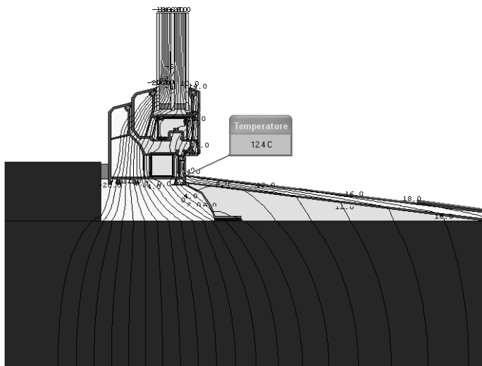
Рисунок К.8 – Температурное поле узла примыкания светопрозрачной конструкции из ПВХ профиля XXXXXXXXXXXXXXXXXX . Сечение узла примыкания вертикального бруска оконной коробки к ограждающей конструкции с четвертью. Откос выполнен ПВХ панелью толщиной 10 мм. Без дополнительного утепления внутреннего откоса. Температура на участке примыкания подоконника к коробке рамы 12,4 °С.
