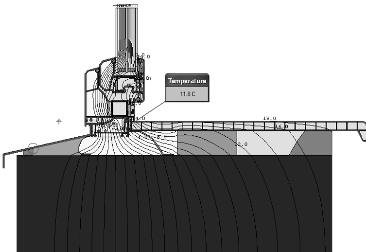
Рисунок К.4 – Температурное поле узла примыкания светопрозрачной конструкции из ПВХ профиля XXXXXXXXXX . Сечение узла в нижней части в зоне расположения опорной колодки ПВХ подоконника. Температура на участке примыкания подоконника к коробке рамы 11,8^{\circ}\text{C} .
