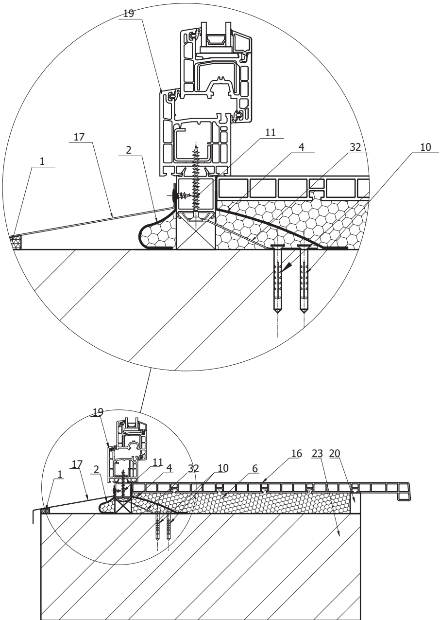
Рисунок А4 – Нижний узел примыкания СПК к проему из штучного материала. Крепление СПК на гибкие анкерные пластины устраняет риск протечки через крепежные отверстия. Лента Робибанд НЛ применена по схеме «внакладку».
