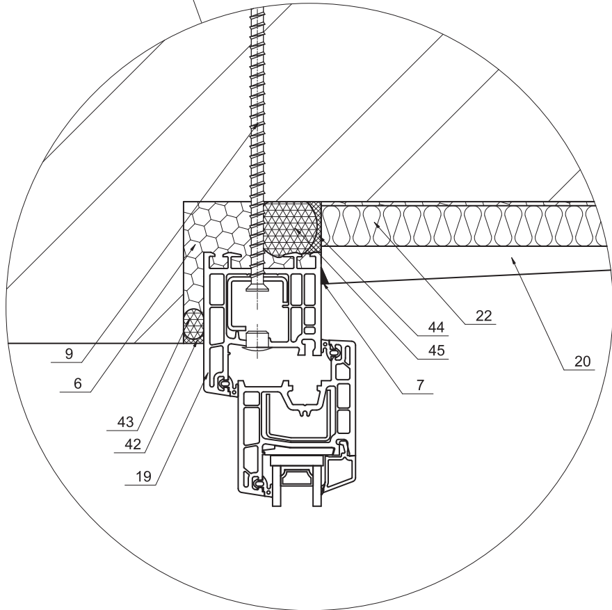
Рисунок А16 – Узел примыкания к проему стены из штучного материала. Проем с четвертью. Внутренние откосы утепляются и оштукатуриваются. Для герметизации монтажного шва применены мастичные герметики.
