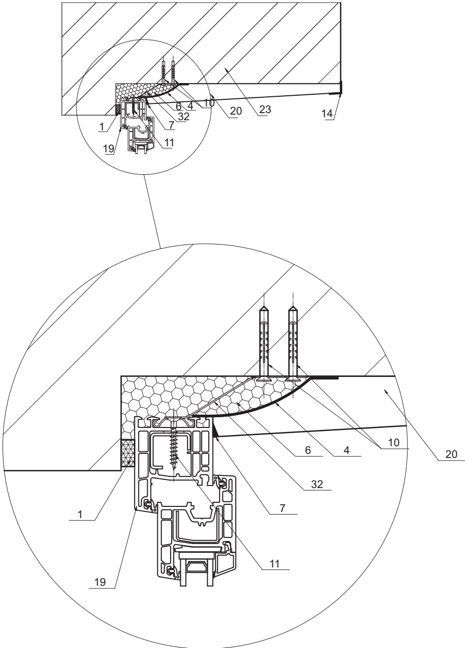
Рисунок А2 – Узел примыкания к проему стены из штучного материала. Проем с четвертью. Внутренние откосы оштукатуренные.
