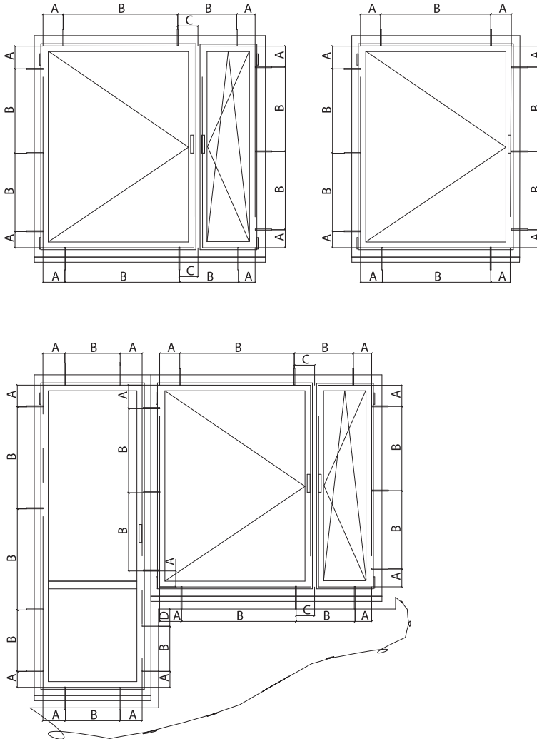
Рисунок Д.1 – Места расположения крепления.
