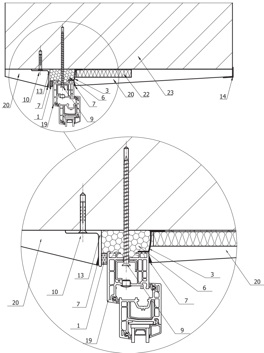
Рисунок А1 – Узел примыкания к проему стены из штучного материала. Проем без четверти. Организация фальшчетверти с применением металлического или пластмассового уголка. Внешние откосы оштукатуриваются. Внутренние откосы утепляются и оштукатуриваются.
